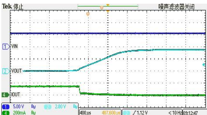
短路释放
