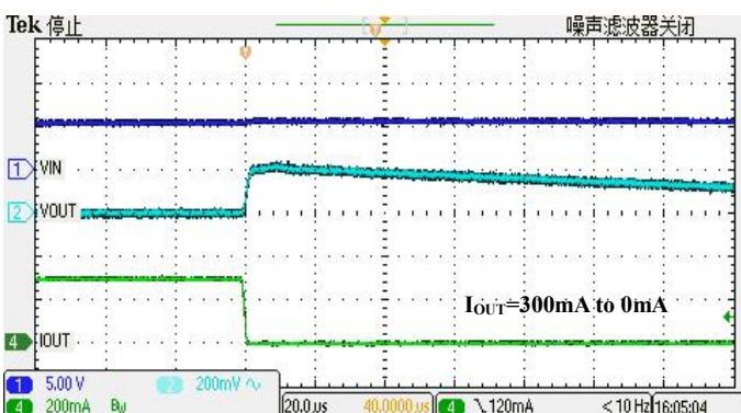
负载跳变
