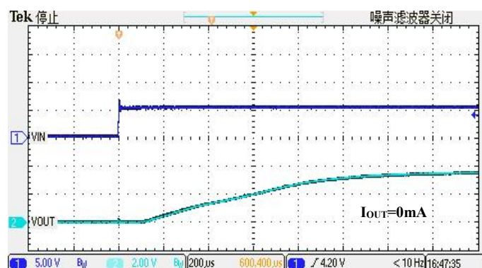
空载上电
