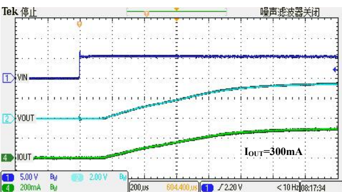
带载上电
