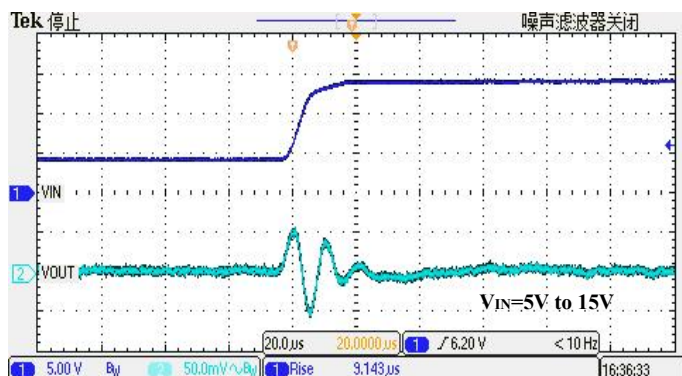
输入跳变
