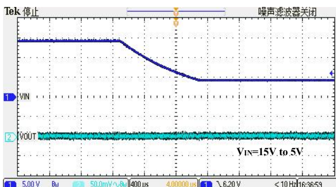
输入跳变
