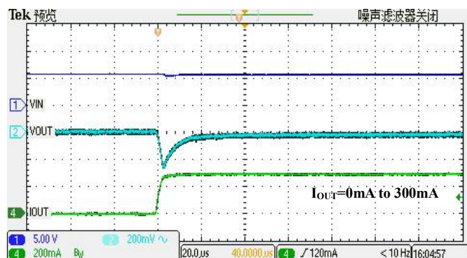
负载跳变
