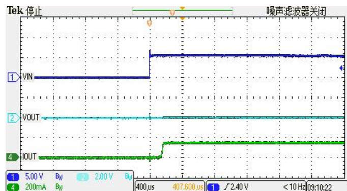
短路上电
